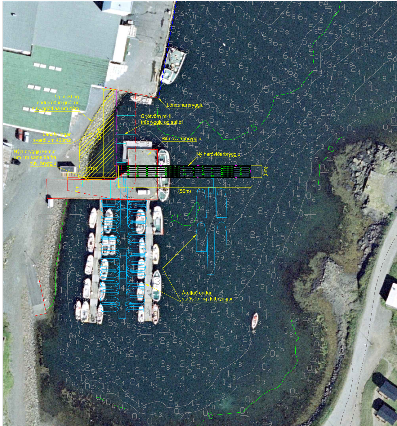
YFIRLITSMYND 1:500
